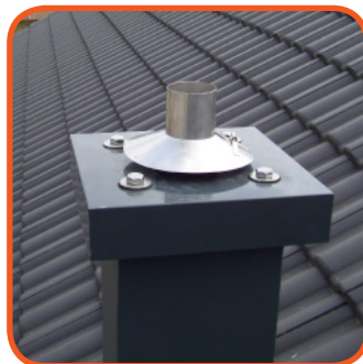
Abdeckplatte Edelstahl lackiert, inkl. Befestigung.
