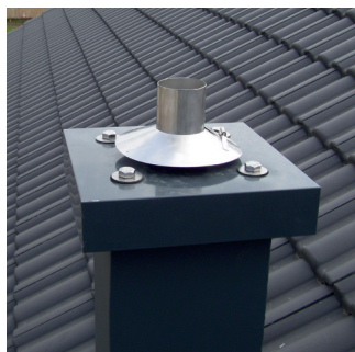
Kopfabschluß 1-zügig: Abdeckplatte Edelstahl lackiert, inkl. Befestigung.
