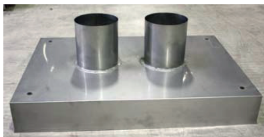
Schornsteinkopfeinfassung Edelstahl Abdeckplatte Edelstahl lackiert, inkl. Befestigung. Nach Maß gefertigt.
