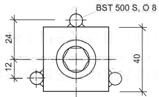
Detail Schnitt A - A
