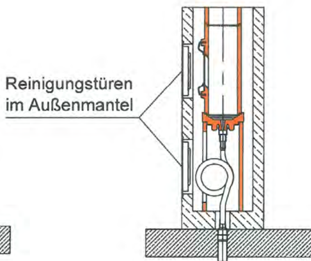
Beispiel der Sockelausführung mit zentralem Kondensatablauf mit Siphonschlauch
