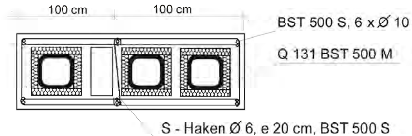
Schnitt A - A bei Schornsteingruppen
