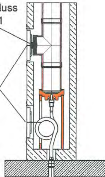
Beispiel der Sockelausführung mit zentralem Kondensatablauf mit Siphonschlauch
