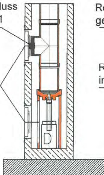
Beispiel der Sockelausführung mit geschlossenem Kondensat - Auffangbehälter
