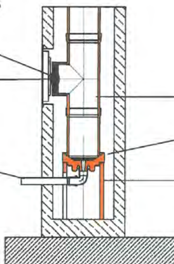
Beispiel der Sockelausführung mit seitlichem Kondensatablauf
